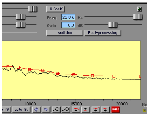
BNR AudioSuite
